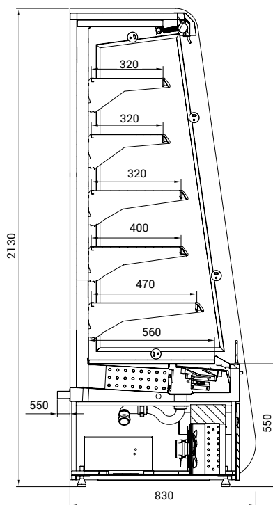
bokorys R Dolce
