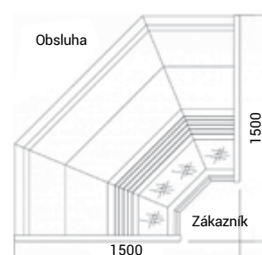
roh 90° uzavřený ventilovaný
