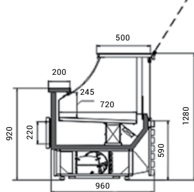
ventilovaná verze PS D Slim
