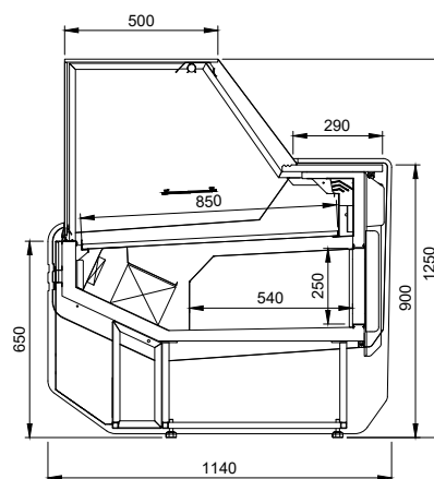
ventilovaná verze W
