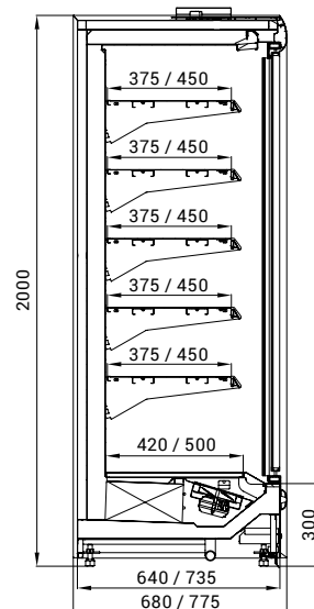
posuvné dveře DP
