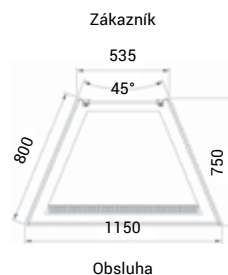
roh 45° uzavřený ventilovaný NW
