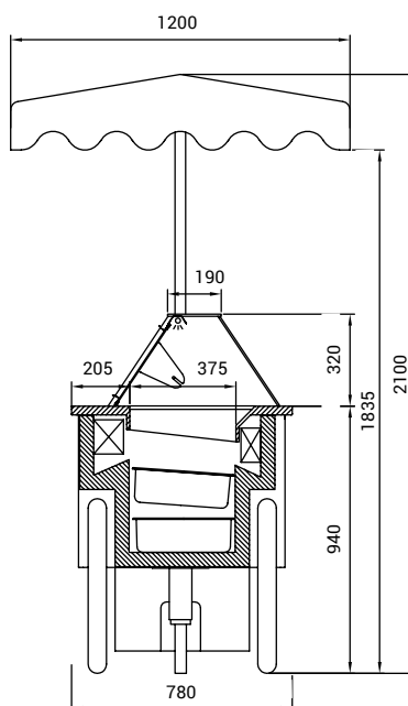
bokorys Riksza
