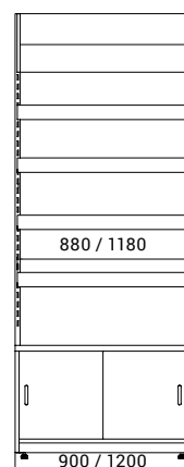
roh 90° otevřený neutrální NZ
