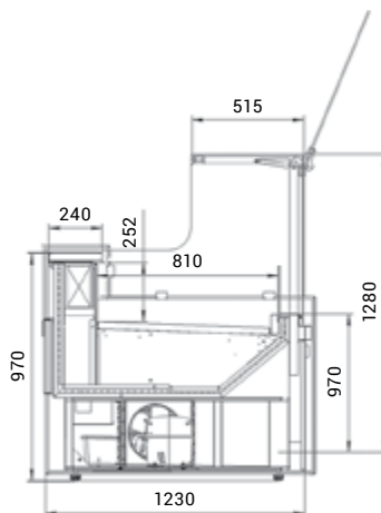
statická verze PS
