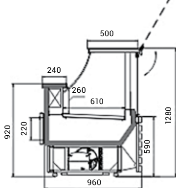
statická verze PS Slim
