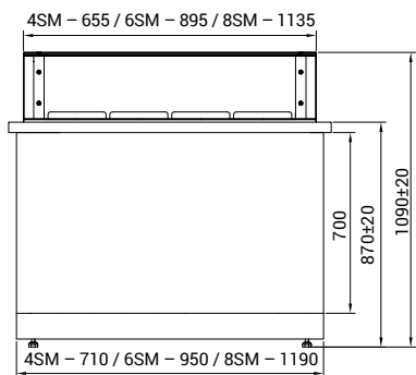
přední pohled
