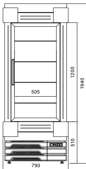
čelní pohled
