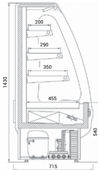
bokorys Piccoli
