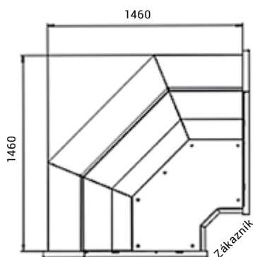
roh 90° uzavřený ventilovaný
