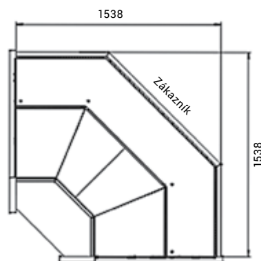
roh 90° otevřený ventilovaný
