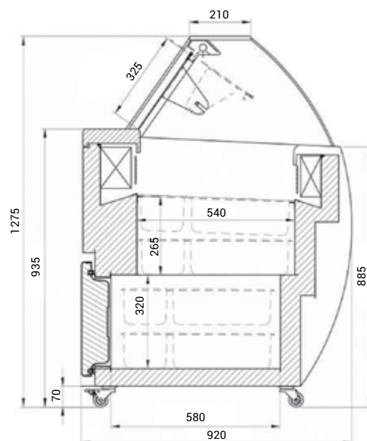
bokorys Tofino KP
