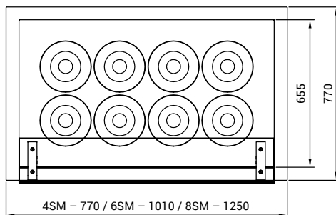
horní pohled
