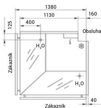
roh 90° otevřený ventilovaný NZ
