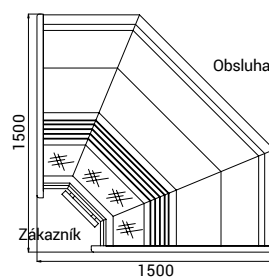
roh 90^{\circ} uzavřený ventilovaný NW
