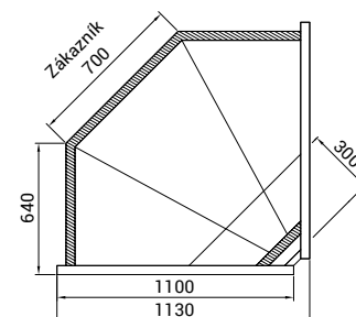
roh 90° otevřený ventilovaný NZ
