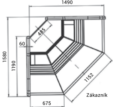
roh 90° otevřený ventilovaný
