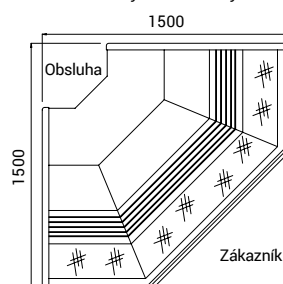
roh 90° otevřený ventilovaný
