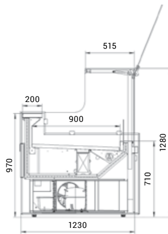
ventilovaná verze PS D
