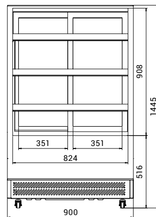
čelní pohled
