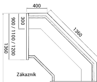
roh 90° uzavřený statický NW
