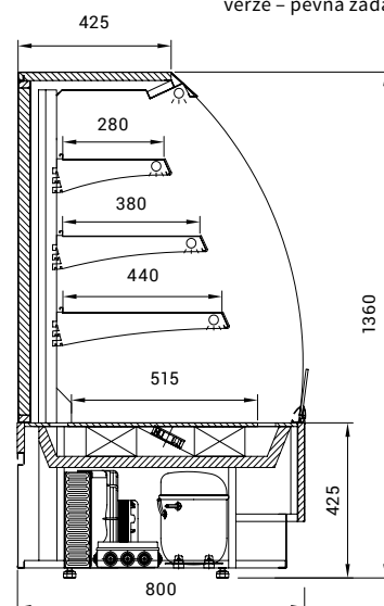
samoobslužná verze – pevná záda
