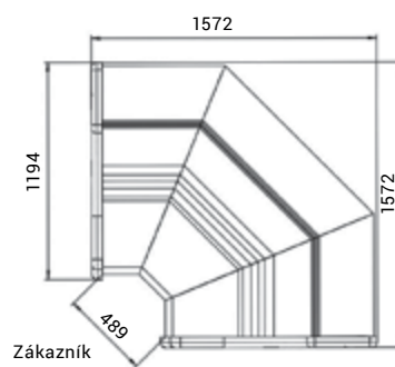
roh 90° uzavřený ventilovaný
