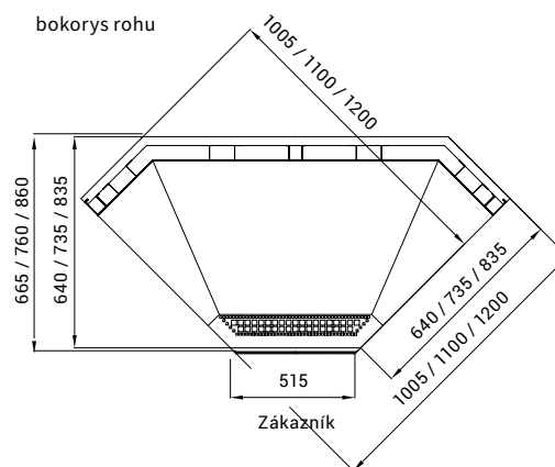
bokorys rohu
