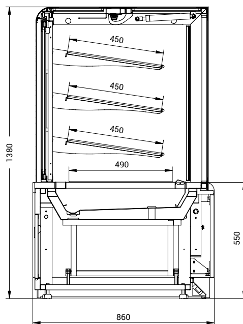
roh 45° otevřený ventilovaný NZ
